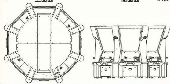
上面図 側面図 1/100
