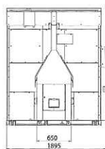
正面図
