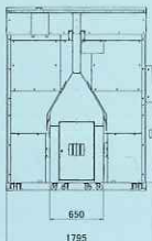
正面図
